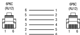
Рисунок 4 – Кабель КС8
